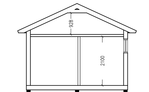
SEKTION A-A
